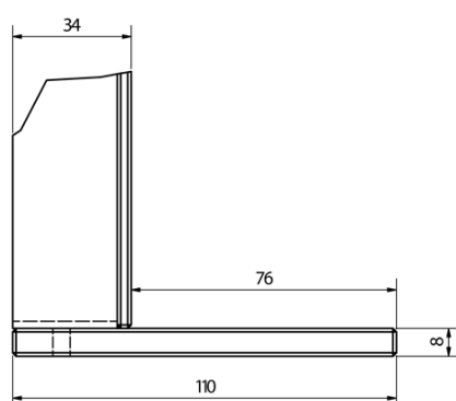
A ( 1 : 1 )
